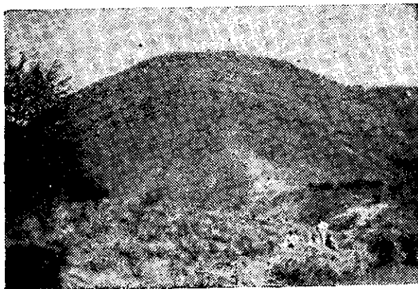
Foto 2) Pendiente oriental del Cerro Aserradero. Arriba: cuarcitas y areniscas compactas, predominantes, de la serie devónica y de la Faja de transición. Abajo: serie arenoso arcillosa amarillenta del Gotlántico fosilífero.
